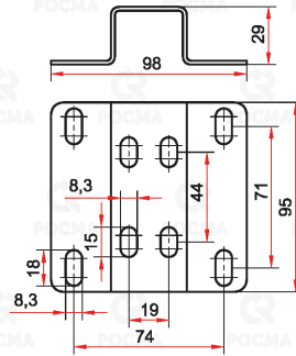
Кронштейн для ТМД-3
